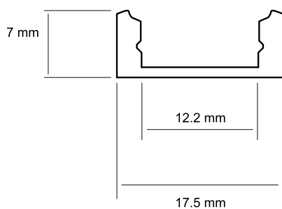
Clip di fissaggio per modular line Mounting clip for modular line
